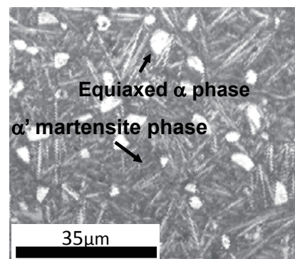
図 1 新しいタイプの ( \alpha + \alpha' ) duplex 組織
